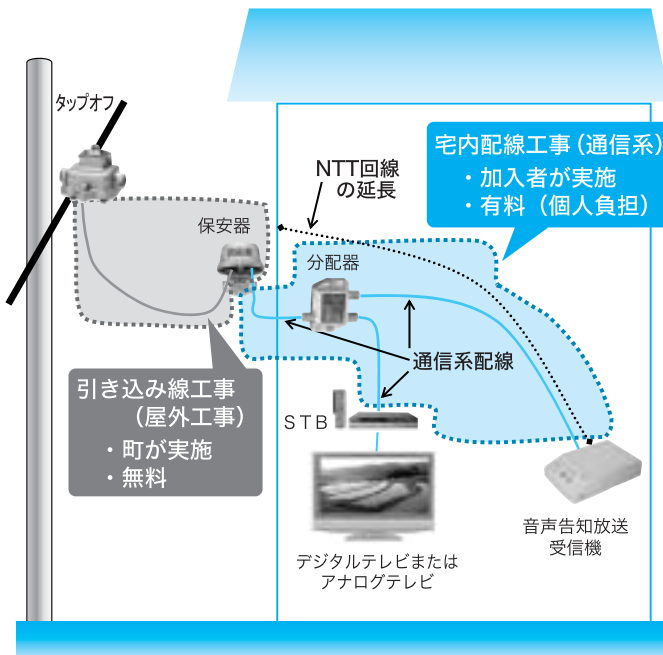
図1 引き込み線工事(屋外工事)と宅内配線工事の区分
