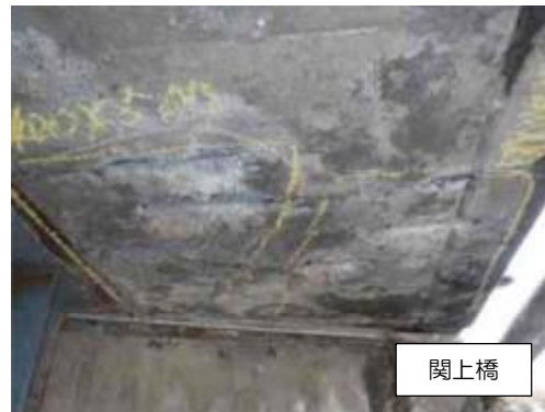
写真 3-3-14 剥離・鉄筋露出
