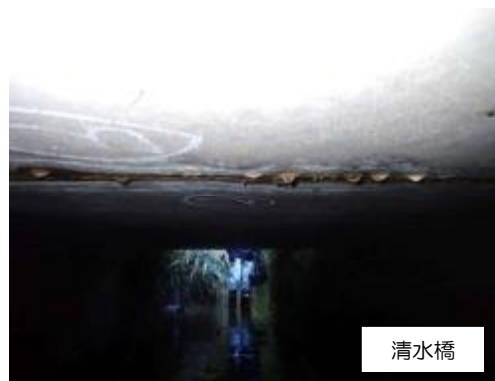
写真 3-3-20 漏水・滞水
