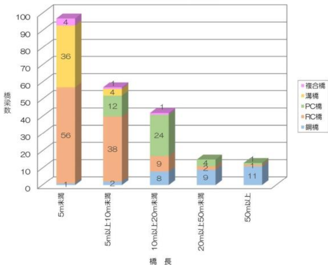
図 2-2-2 橋長の分布
