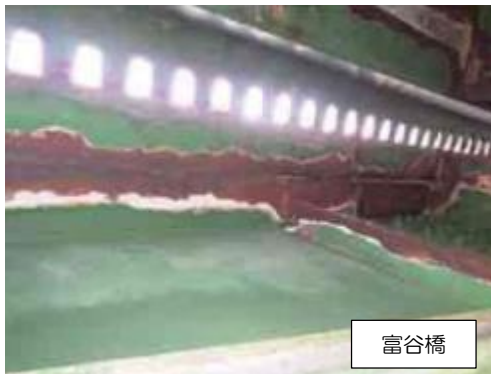
写真 3-3-25 腐食(1)
