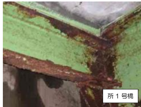
写真 3-3-26 腐食(2)
