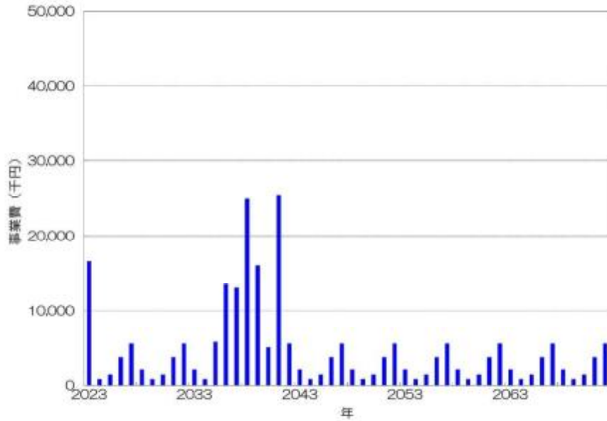
図 4-5-3 事業費用の推移 (個別 LCC : グループ B)
