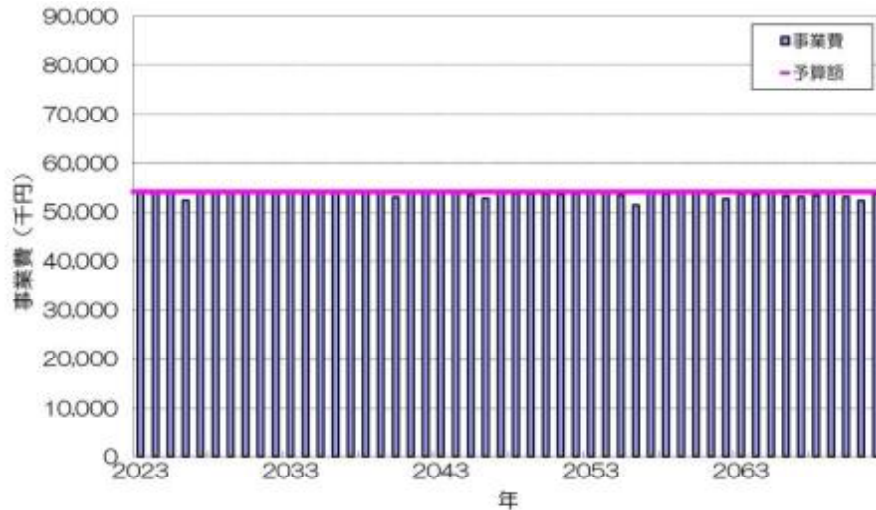
図 4-5-8 事業費用の推移（制約 LCC：年予算 5,400 万円）
