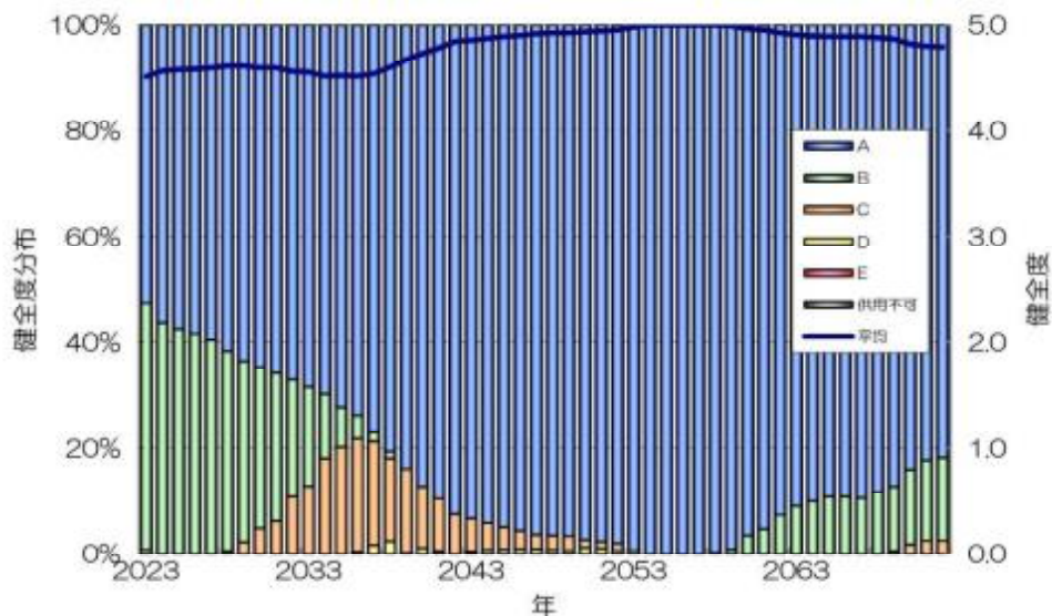
図 4-5-11 健全度分布の推移
