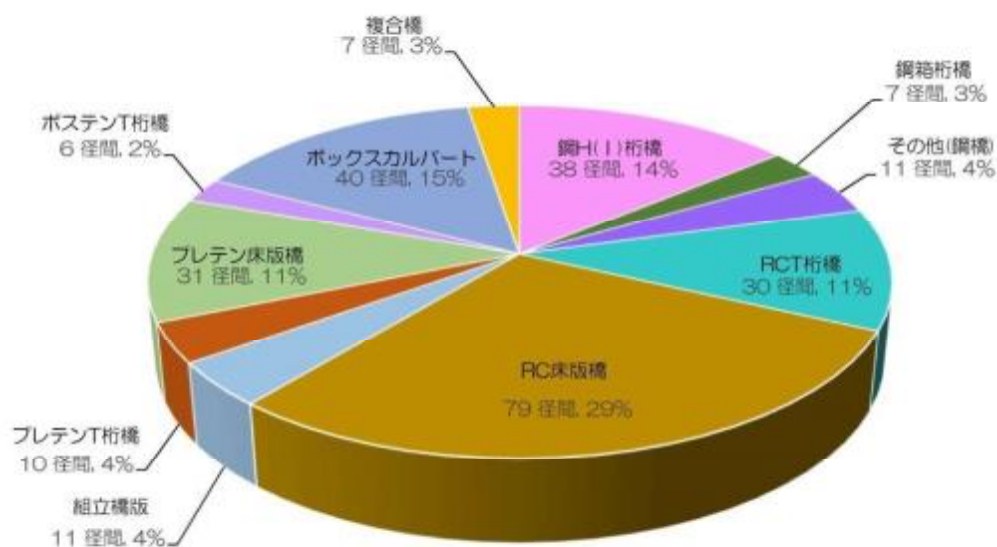
図 2-2-5 構造種類別径間数
